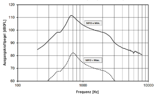
Telefonspulencharakteristik
