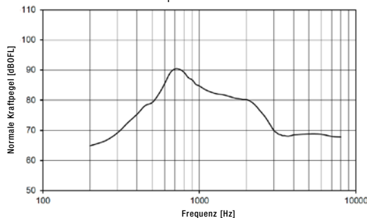
Telefonspulencharakteristik
